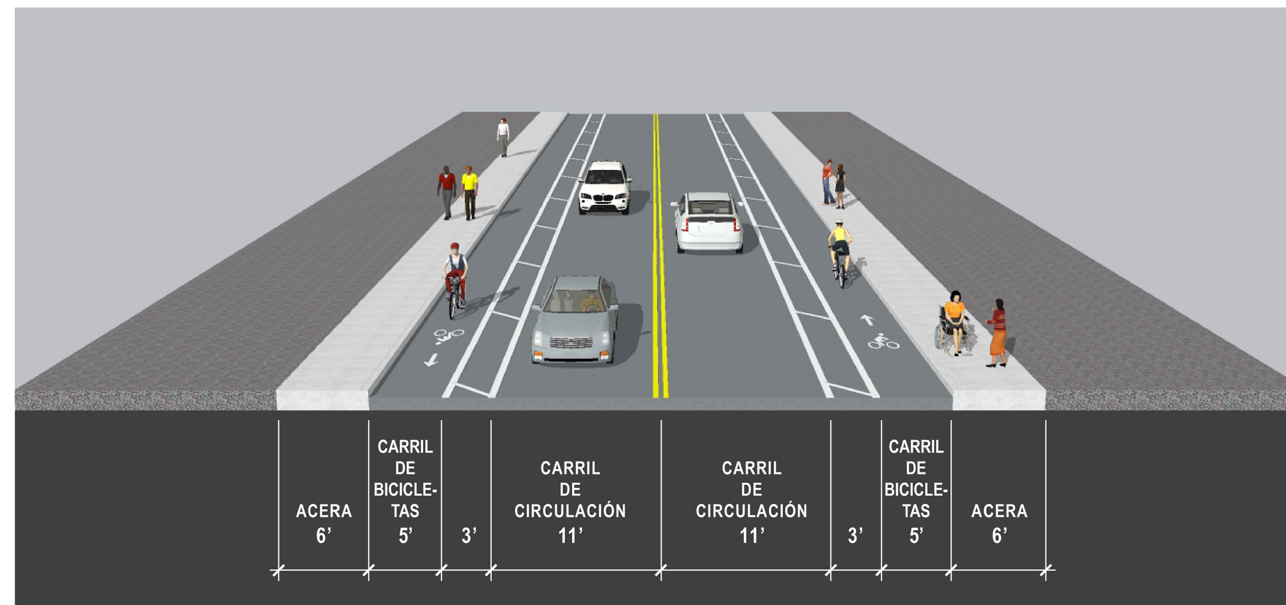
Dos Carriles de Circulación sin una Tira de Paisajista
