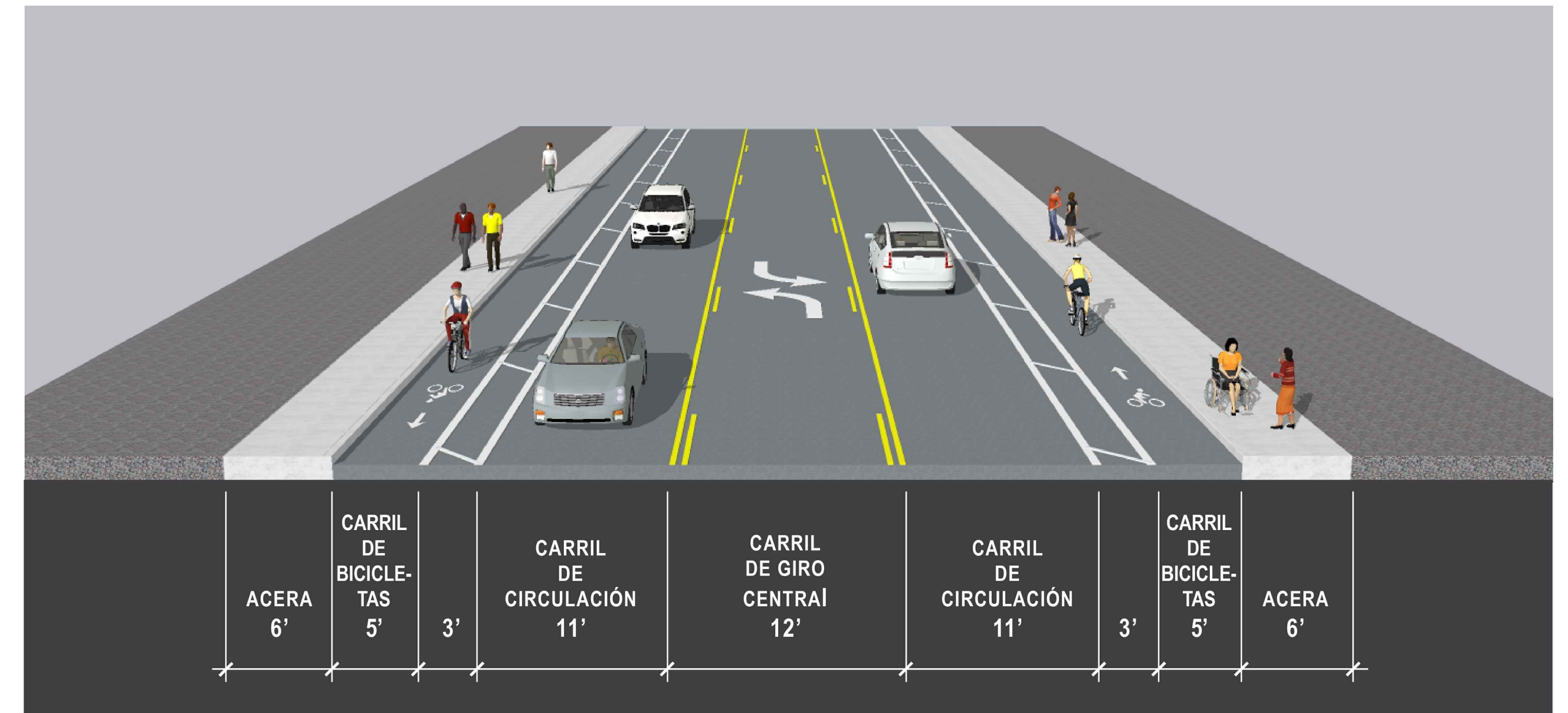
Tres Carriles de Circulación sin una Tira de Paisajista
