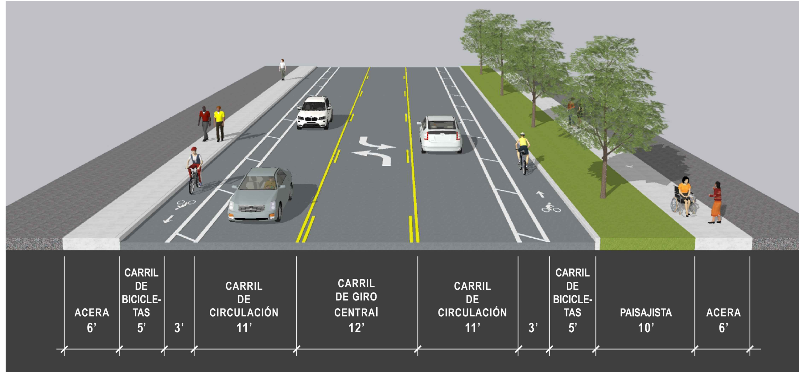
Tres Carriles de Circulación con una Tira de Paisajista
